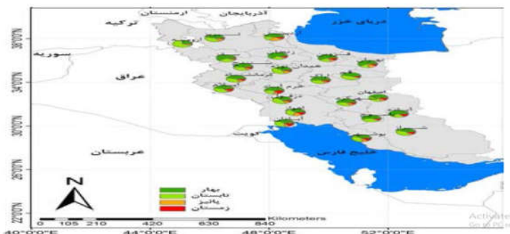
نقشه (۲). توزیع فصلی فراوانی وقوع پدیده گرد و غبار برای هر یک از ایستگاه‌های واقع در نیمه غربی ایران (عزیزی و میری، ۱۳۹۱: ۹)
