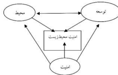
شکل (۱). نسبت امنیت با محیط‌زیست (کاویانی راد، ۱۳۹۰: ۹)
